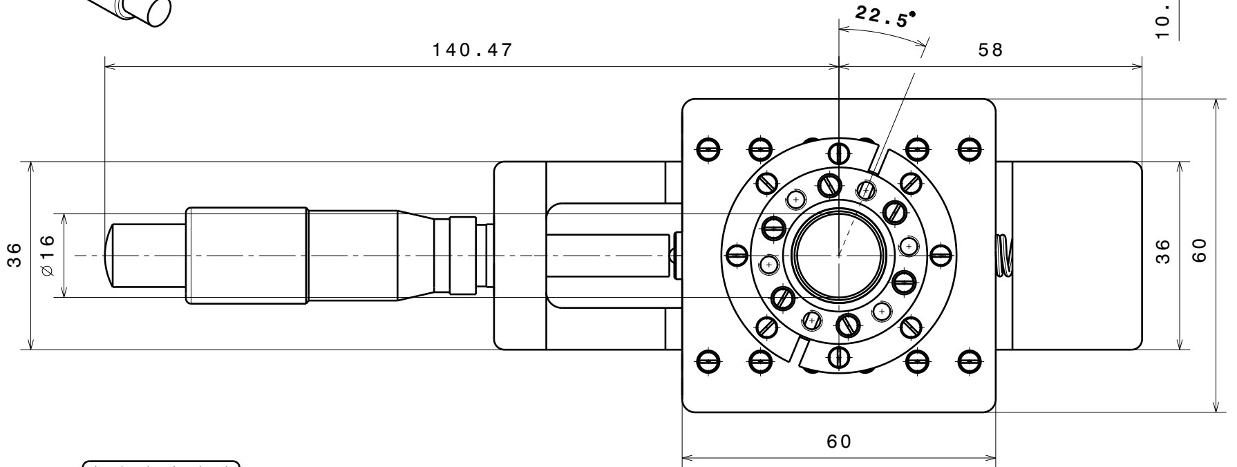
Rückansicht Maßstab: 1:2
